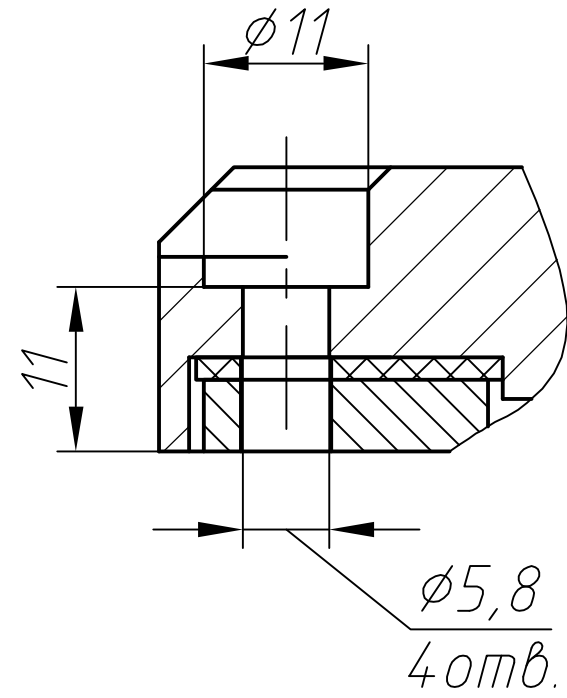
Б-Б (1:1)
