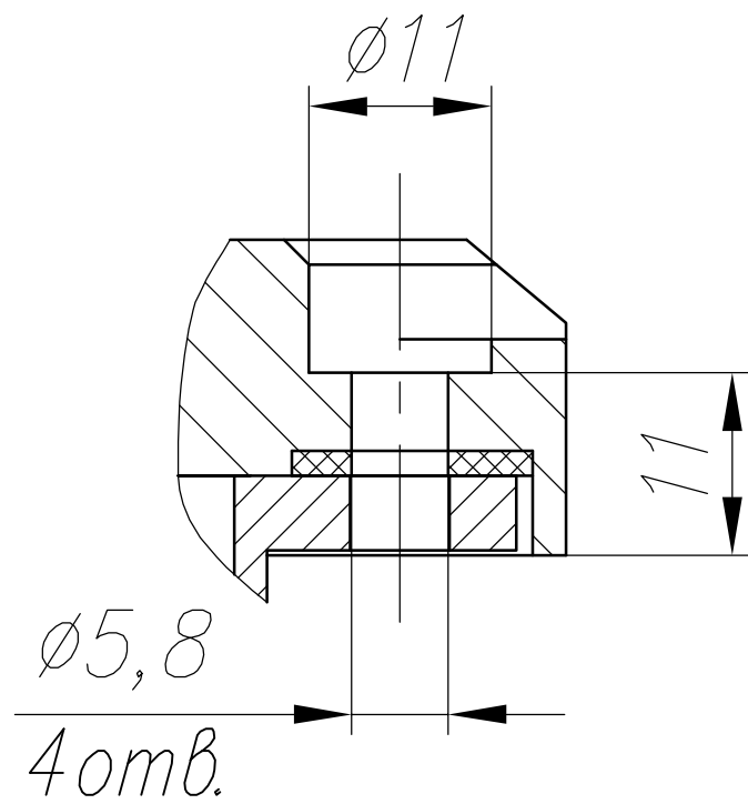
B-B(1:1)
