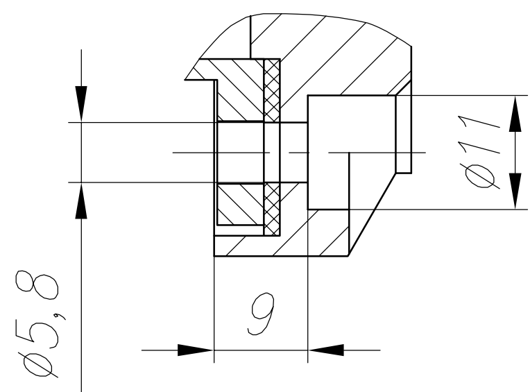
B-B(1:1)
