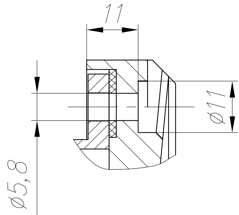
A-A(1:1)
