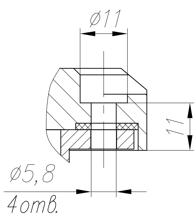
Б-Б(1:1)
