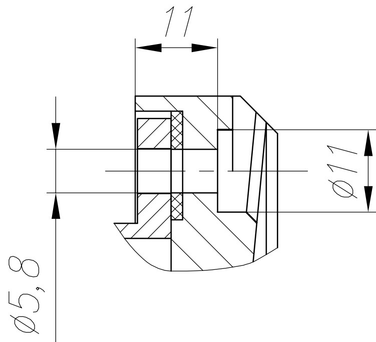
A-A(1:1)
