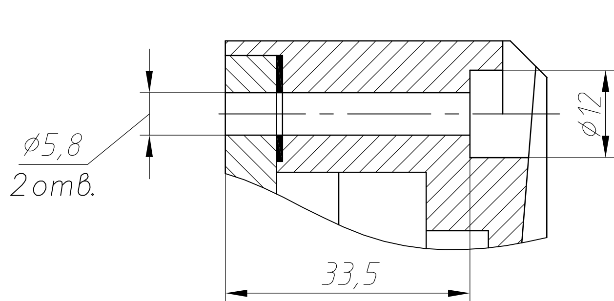
Б—Б(1:1)
