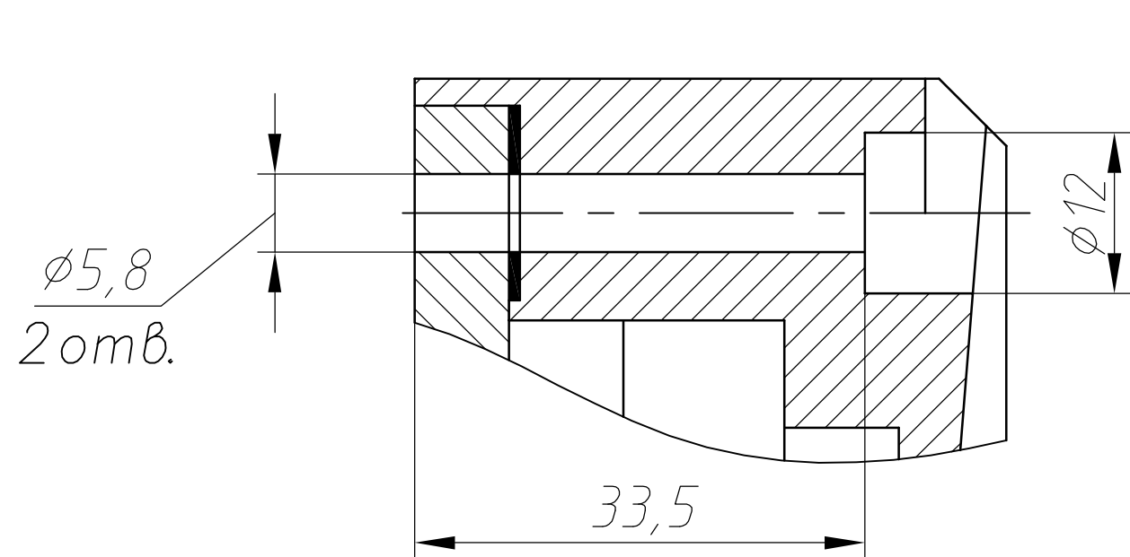
Б—Б(1:1)
