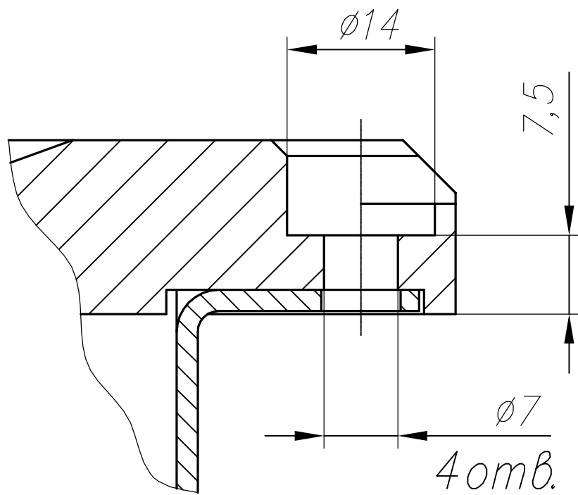
Б-Б (1:1)
