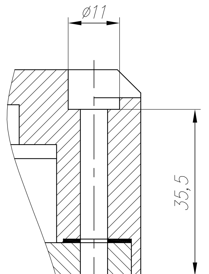
B-B(1:1)
