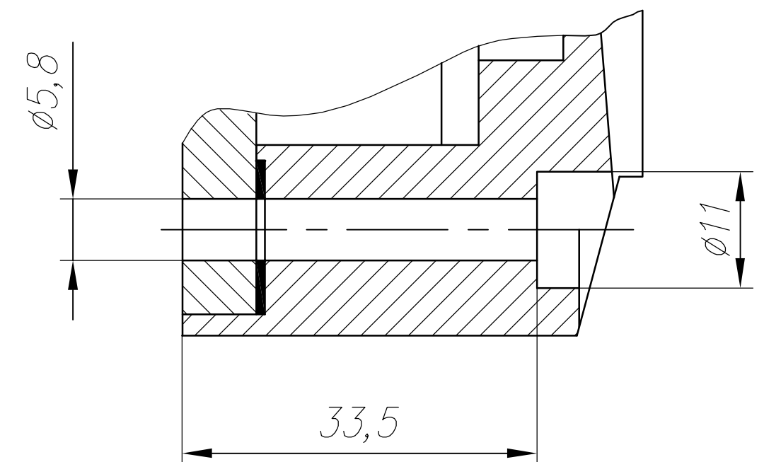
B-B(1:1)
