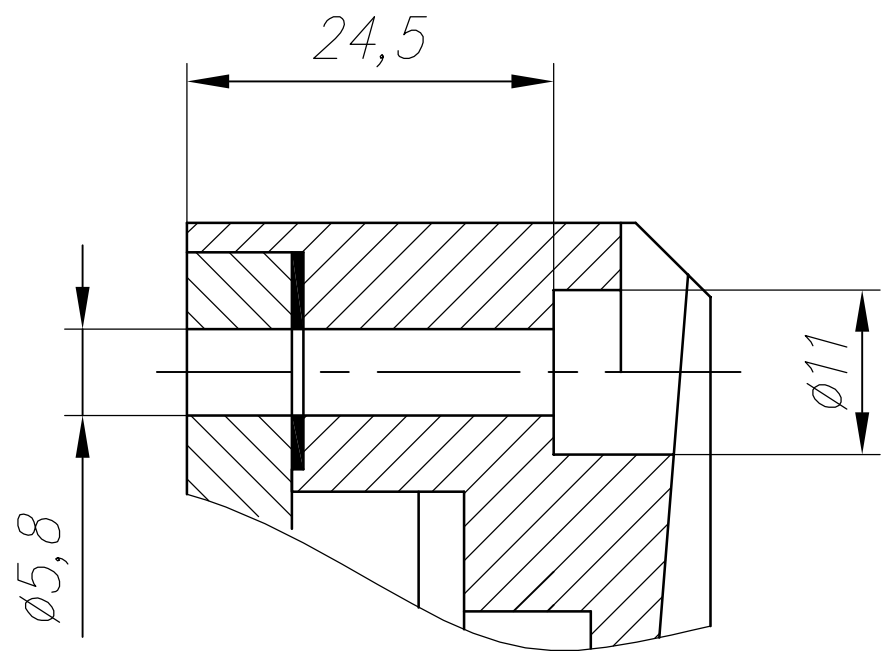
A-A(1:1)
