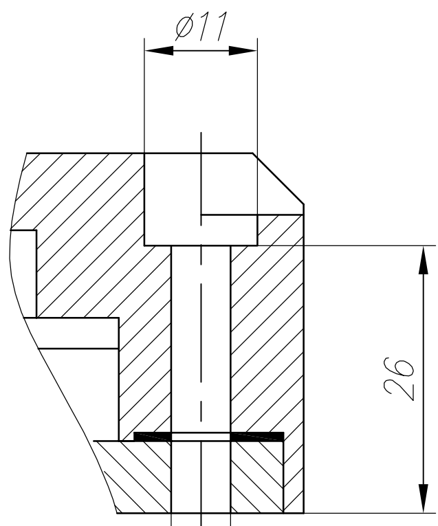
Б-Б(1:1)
