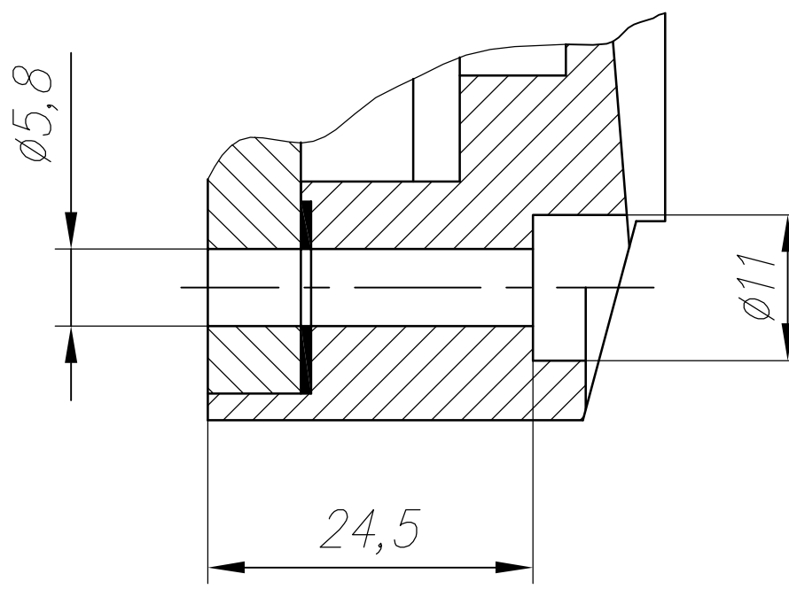
В-В(1:1)
