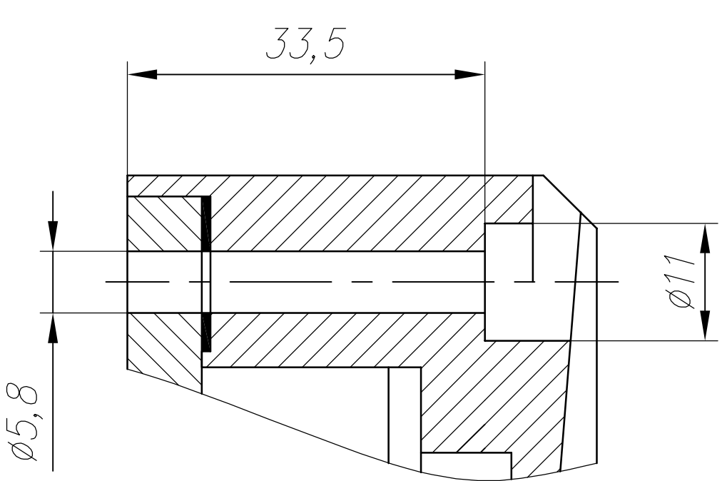
A-A(1:1)
