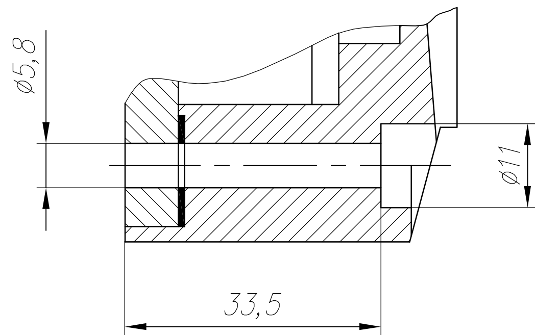
B-B(1:1)
