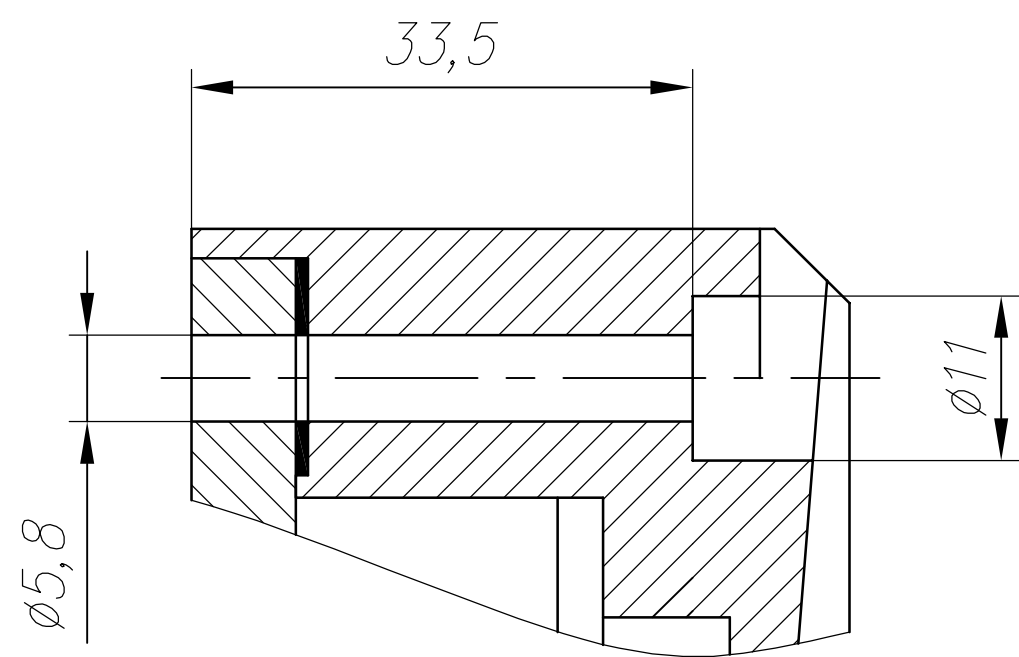
A-A(1:1)
