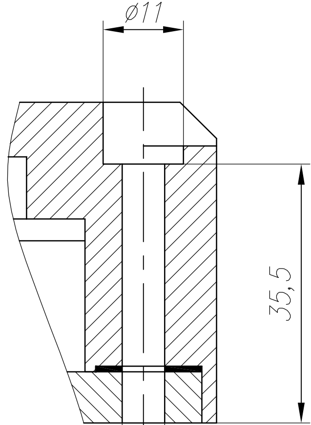
B-B(1:1)
